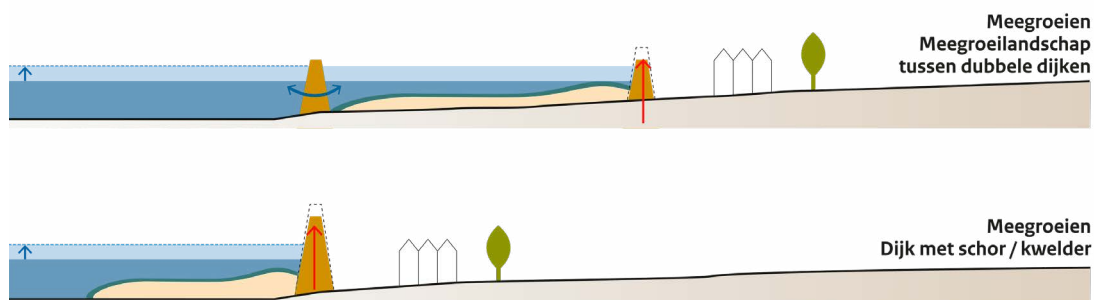
Figuur 1b: Dwarsdoorsnede van twee mogelijke bouwstenen uit de denkrichting Meegroeien. In beide gevallen zal de achterliggende dijk in de toekomst minder versterkt hoeven te worden dan zonder aanslibbing.
