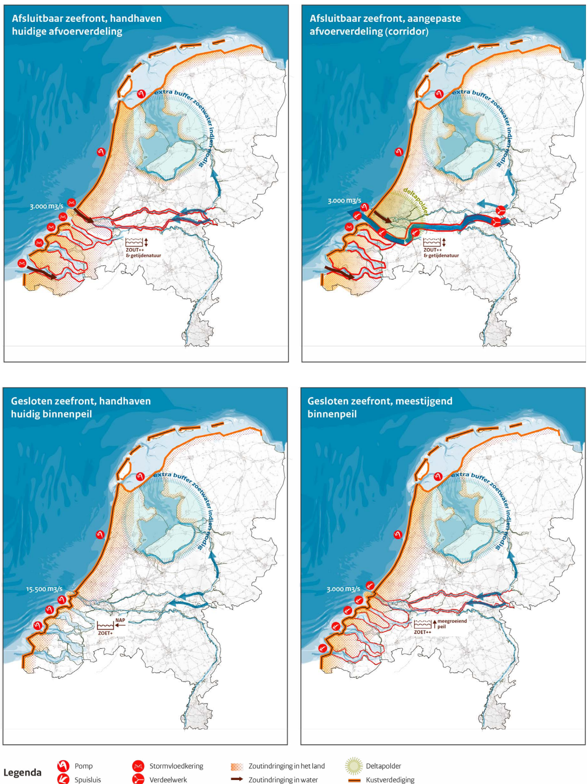
Figuur 4: De onderzochte 4 strategieën van de denkrichting Beschermen: afsluitbaar zeefront met stormvloedkeringen, meestijgend waterpeil en al dan niet aangepaste afvoerdividing Rijntakken. En gesloten zeefront met hetzij pompen en een laag waterpeil, of spuien en een meestijgend waterpeil om overtollig rivierwater naar zee af te voeren. Door de verschillende combinaties van bouwstenen verschillen de strategieën in optredende verzilting en benodigde dijkversterkingen.
